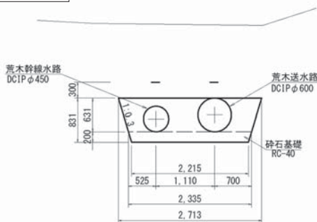
標準断面図
